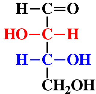
D-Threose
