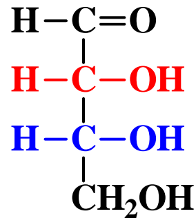
D-Erythrose
