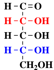
D-Ribose
