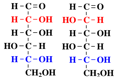
D-Gulose
