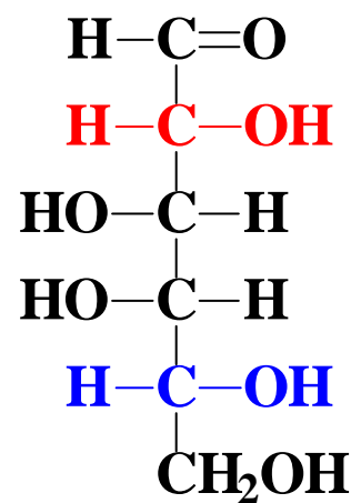
D-Galactose
