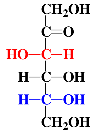
D-Fructose
