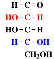
D-Lyxose
