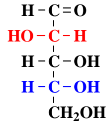
D-Arabinose
